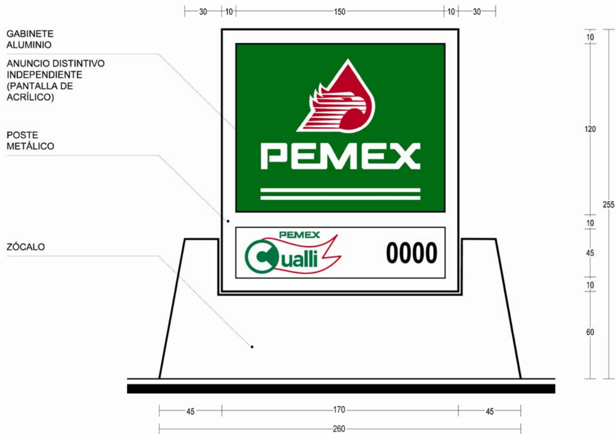
ALZADO FRONTAL
